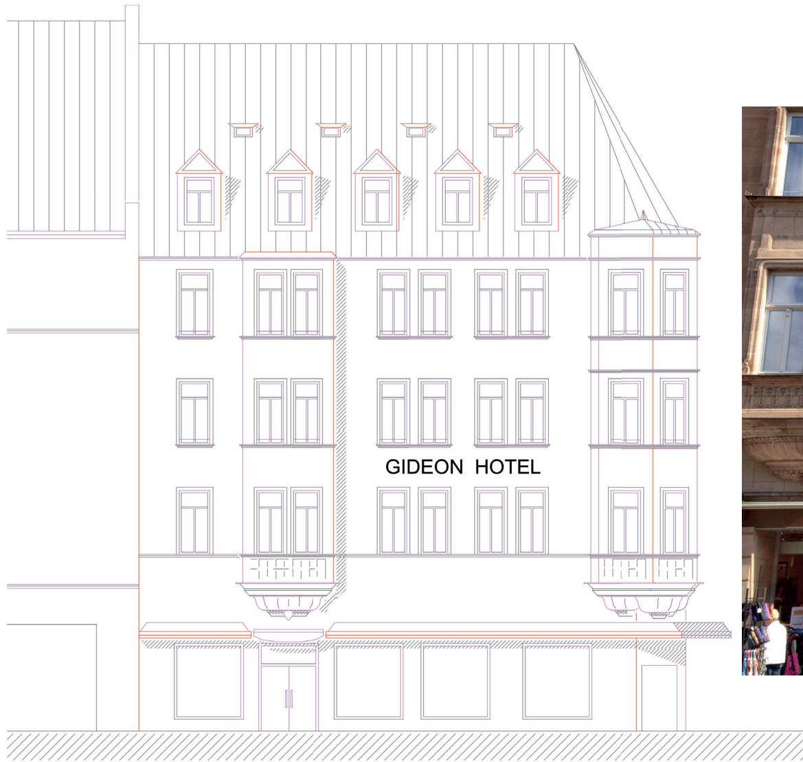
Ansicht Südwest/Königstrasse
