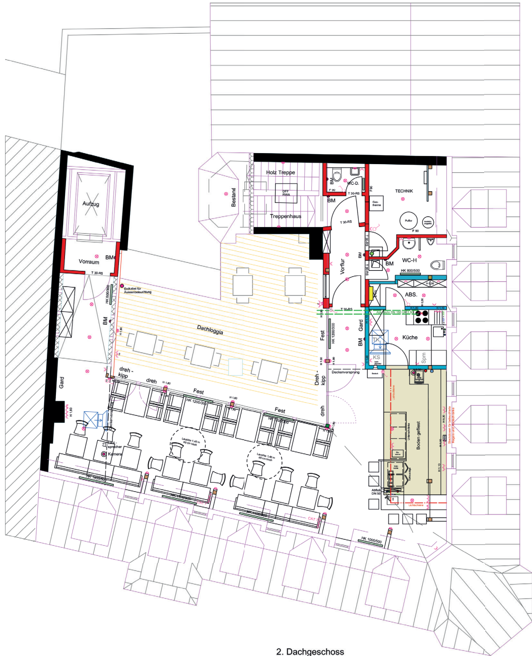
2. Dachgeschoss
