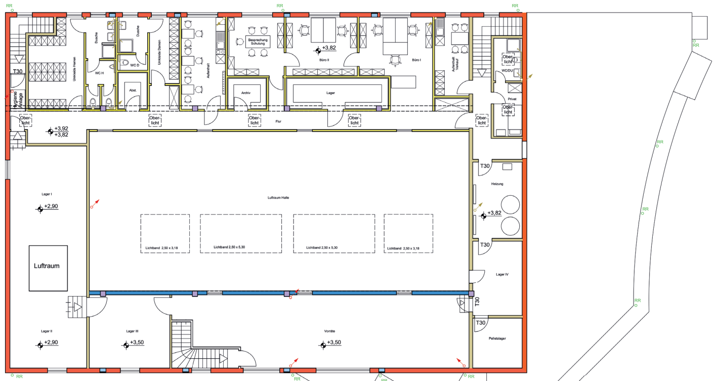
Obergeschoß
